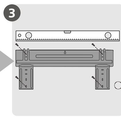
Kiinnitä kiinnityslevy
